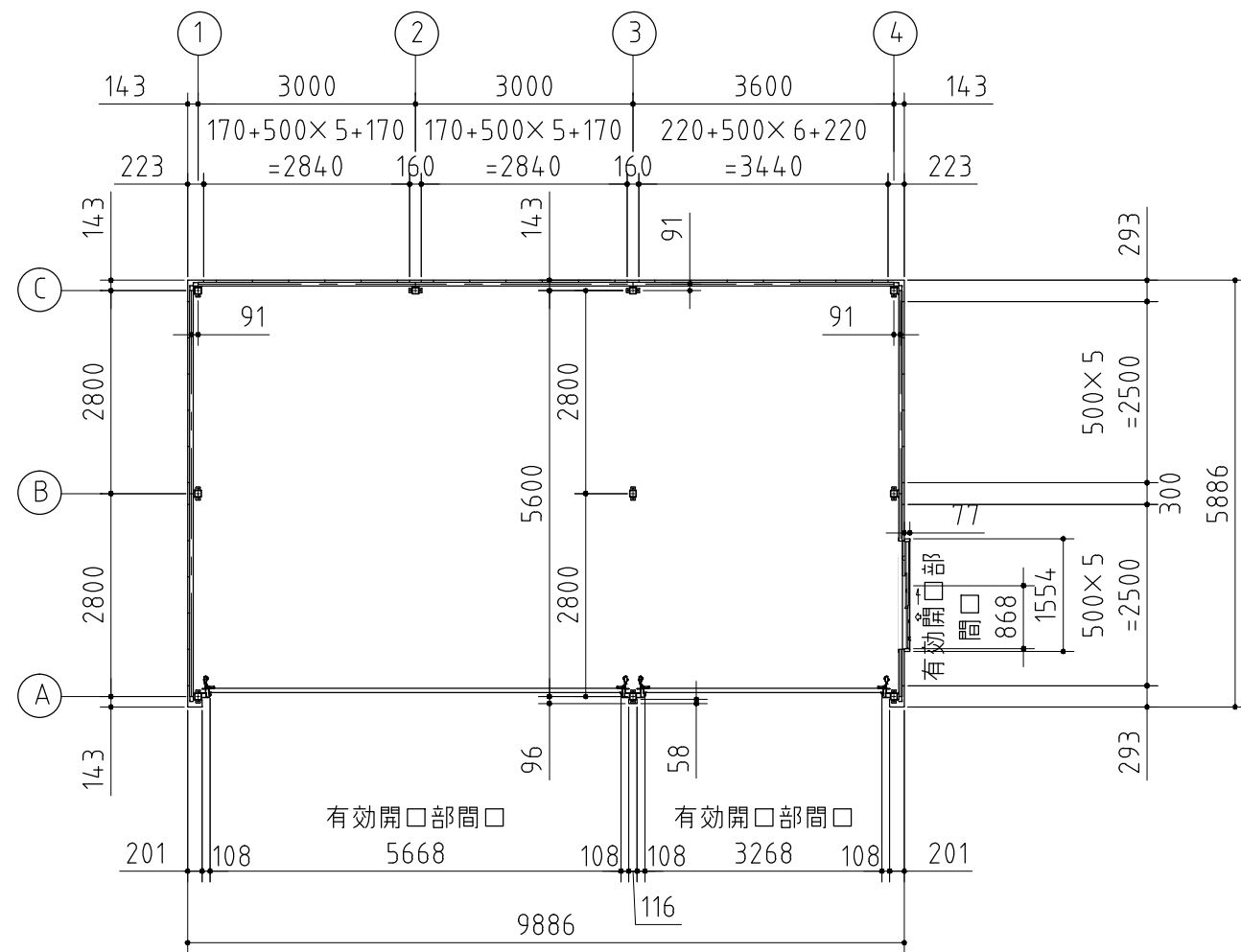
平面図
